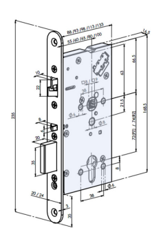
Serrure porte standard
