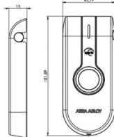
Electronique extérieure (tête de lecture)
