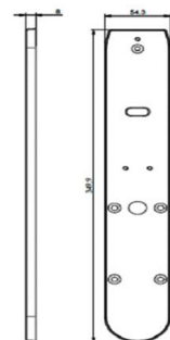
Plaque extérieure (si commandée)
